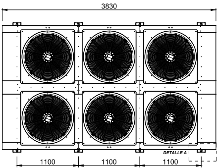
VISTA LATERAL
